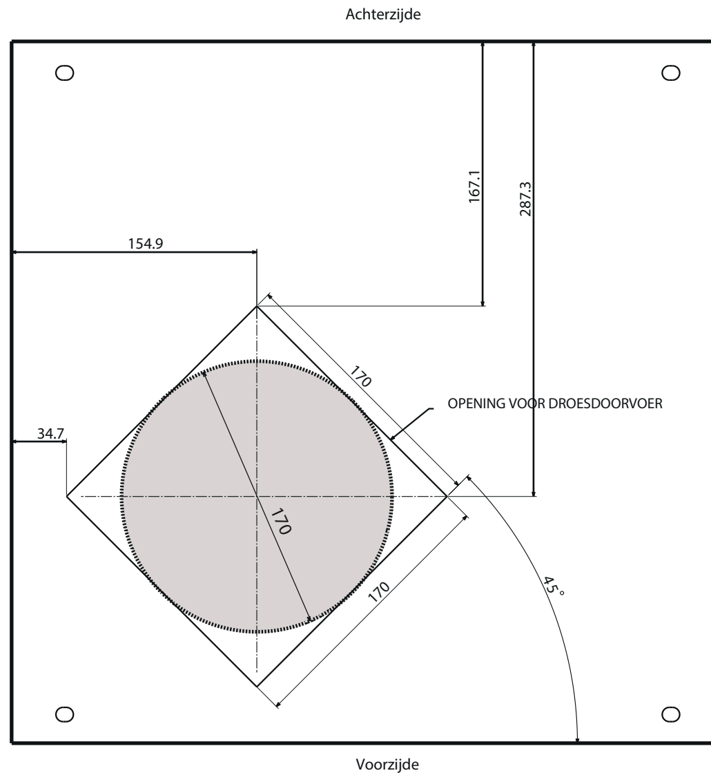
MACHINE BOVENAANZICHT
