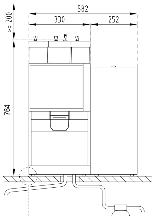
Voorzijde machine
