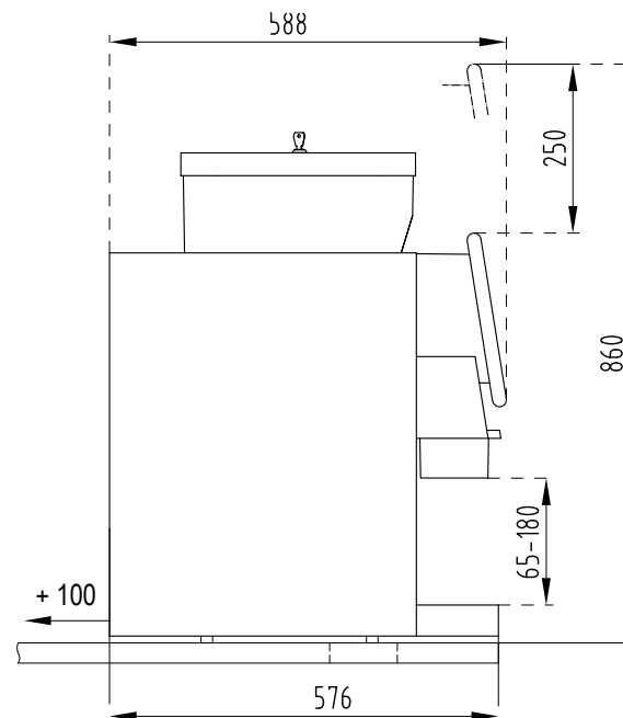
Zij-aanzicht machine
