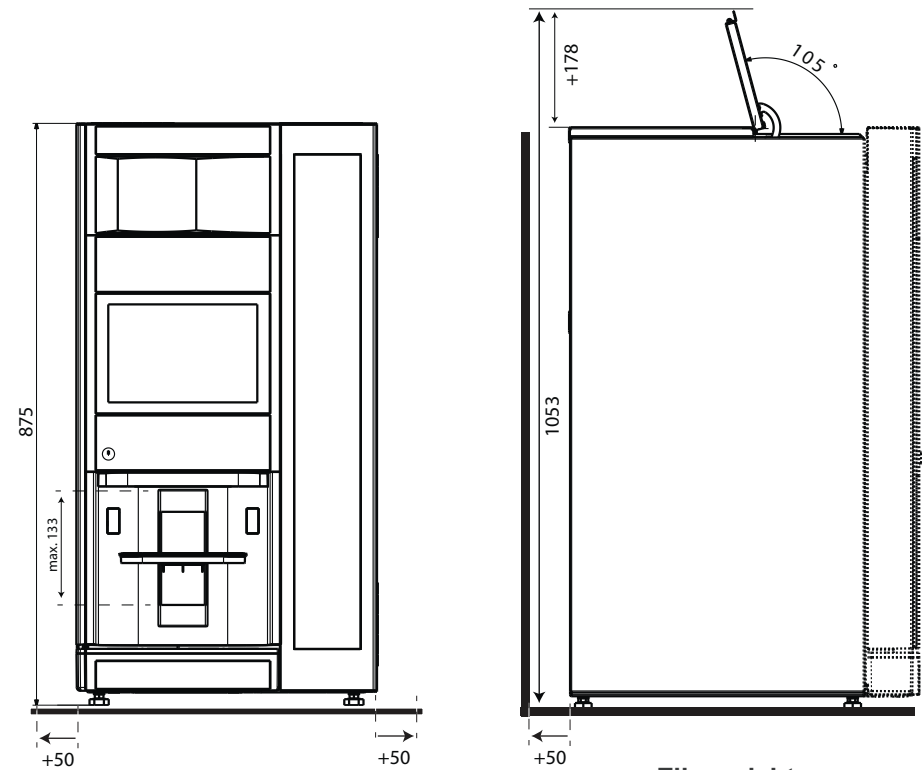
< Zijaanzicht >
