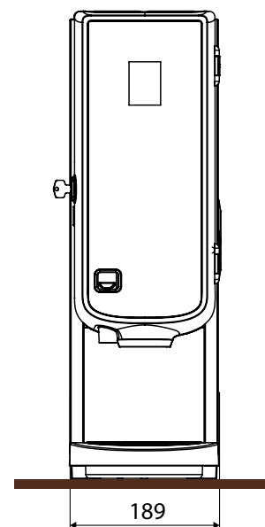
Voorzijde (100 mm aan beide zijden t.b.v. service en ventilatie)
