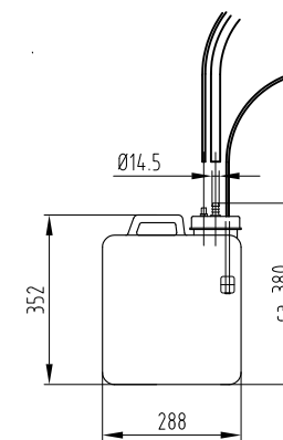
Vuil-water tank 13L
