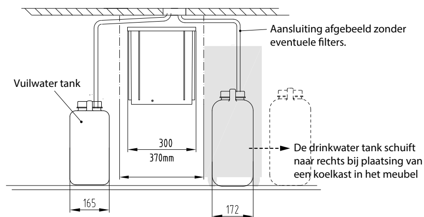
Vuil-water tank 13L
