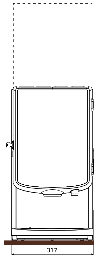
Voorzijde (100 mm aan beide zijden t.b.v. service en ventilatie)
