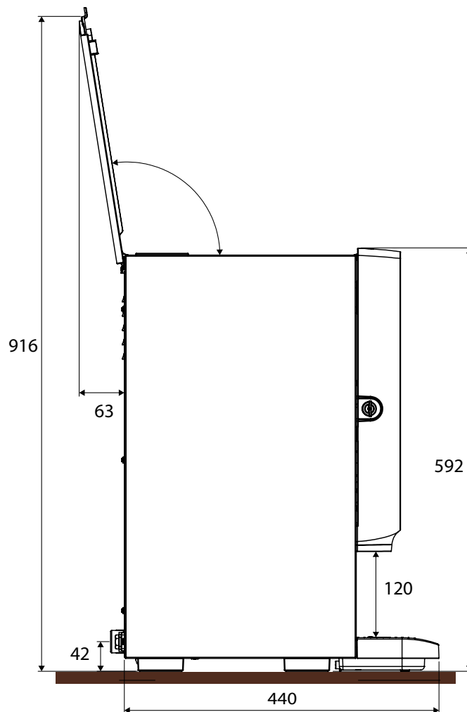
Zijkant met geopend bovendecksel (+80 mm ruimte aan de achterzijde)
